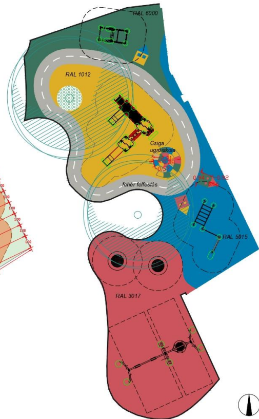
EPDM réteg
