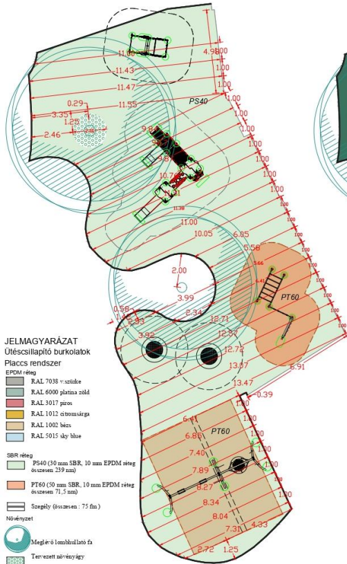
SBR réteg
